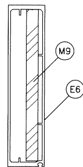
JAMB 'J2'
