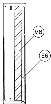
JAMB 'J3'
